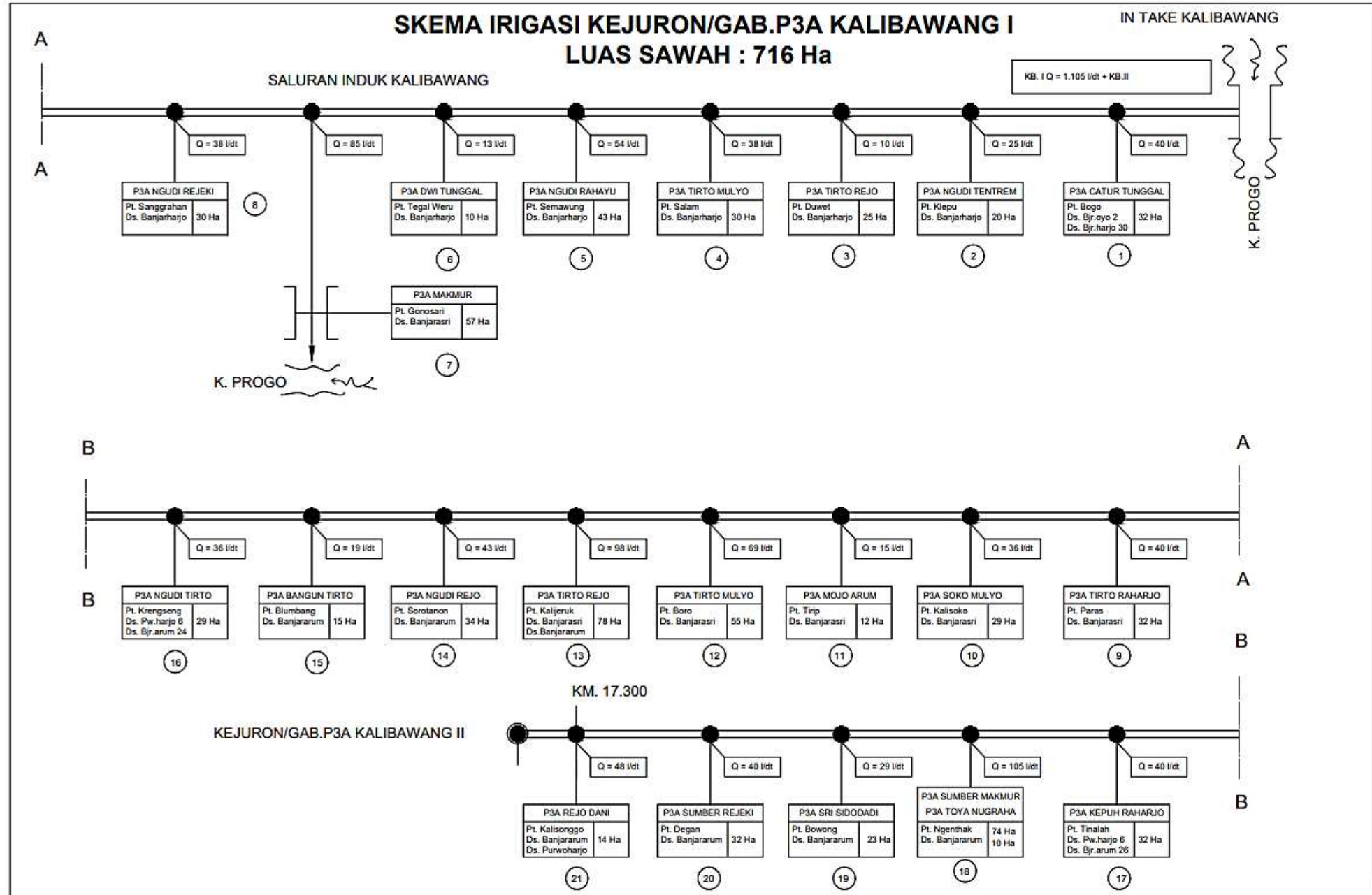
A. SKEMA IRIGASI KEJURON PENGAIRAN
